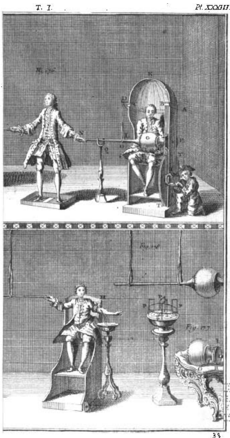
Slika 7: Naelektrotev izoliranih oseb po Slovarju Alexandra Saveriena, ki ga je uporabljal Hal- lerstein (Saverien, Dictionnaire universel de mathématique et de physique , tabla 43).
