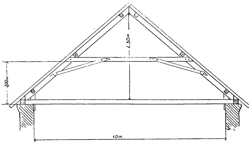
Sl. 8. Pibrovec (h. št. 82). — Strešni stol
