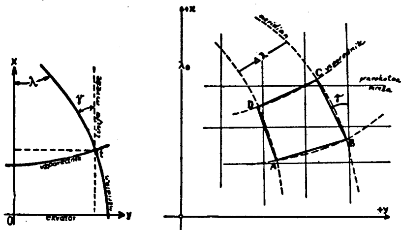
Slika 2 a in b. Projekcija kartnega izreza A B C D na zemeljskem obodu v projekcijsko ravnino. Kot odklona y stvarnega zemeljskega meridiana od projekcijske mreže je t. i. meridianska konvergenca.
