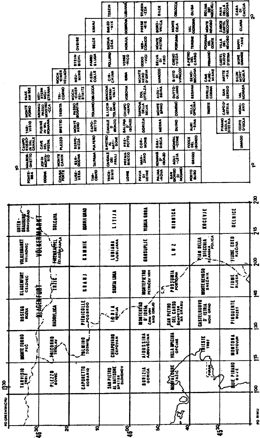
Slika 16. Shema listov dopolnjene nemške izvedene karte ITALIEN 1:50 000 (levo) in 1:25 000 (desno) iz 1944/45.
