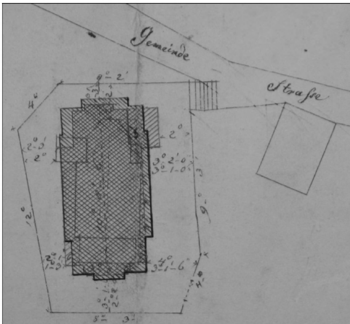
Situacija stare cerkve z variantnima načrtoma nove cerkve iz leta 1860 (ARS, AS 140, mapa 2).
