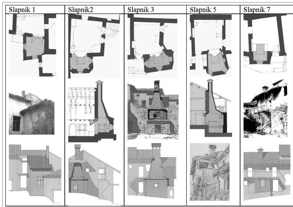
Dokumentirane spahnjenice v Slapniku (izris: Aleš Princič, 1983).
