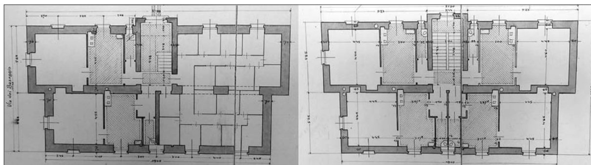
Tloris pritličja in kleti (levo) ter zgornjih nadstropij (desno) večnadstropne stavbe ob via Baseggio (G. B. Finetti, 1906) (ATD – Ts, načrt št. 8809).
