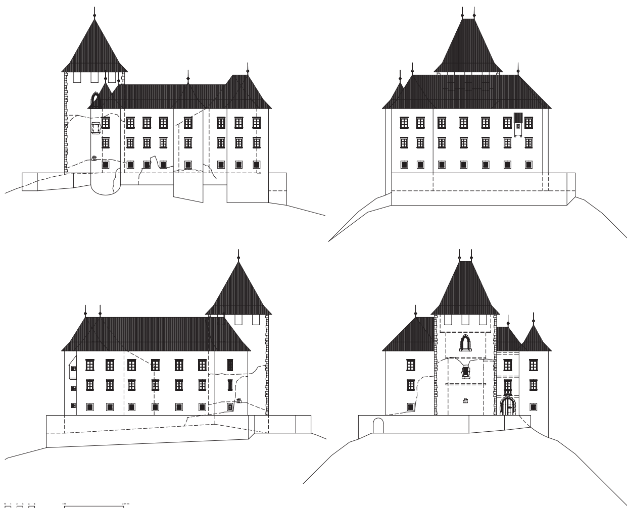
Poskus rekonstrukcije oblike zunanjih fasad gradu Rudenek oziroma njegovega severovzhodnega dela v prvi polovici 17. stoletja (risal: Igor Sapač, 2024).
