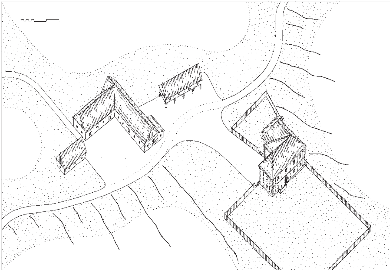
Dvor(ec) Lešje v 17. stoletju. Poskus rekonstrukcije. Aksonometrična študija (risal: Igor Sapač, 2025).
