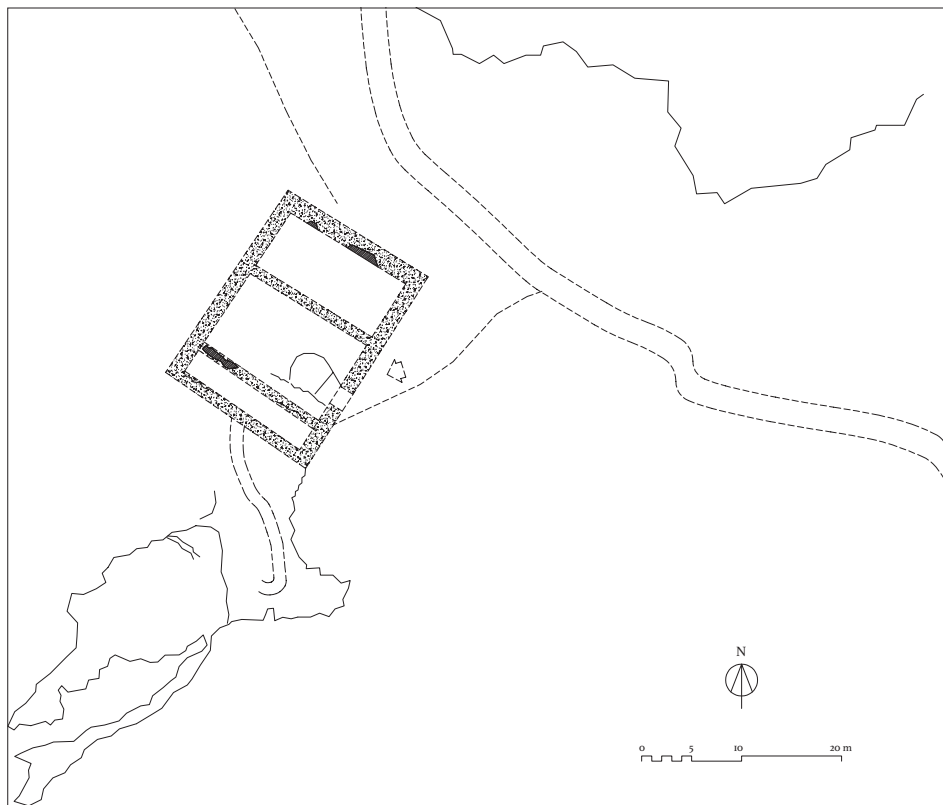
Tloris nekdanjega gradu Rudenštajn s črno označenimi ostanki zidovja v jedru (risal: Igor Sapač, 2025).
