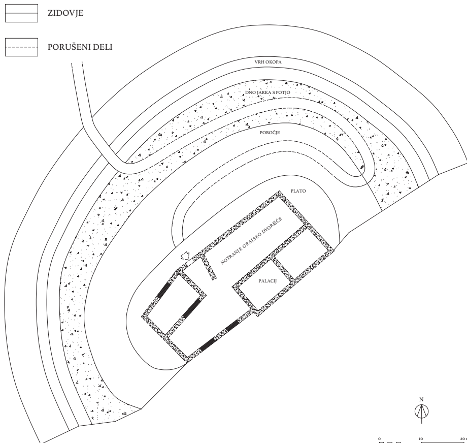
Tloris jugozahodnega dela nekdanjega rudeneškega grajskega kompleksa z obrambnim okopom in jarkom ter s črno označenimi ostanki zidovja grajskega jedra (risal: Igor Sapač, 2024).
