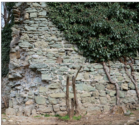
Pogleda na značilno kompartmentno strukturo zidave iz 14. stoletja na jugozahodni (levo) in jugovzhodni stranici (desno) gotskega stolpa gradu Rudenek (foto: Igor Sapač, 2024).
