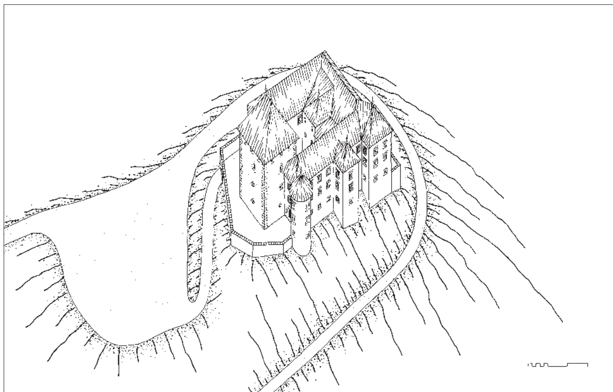
Severovzhodni del gradu Rudenek z gotskim stolpom in renesančno širitvijo v prvi polovici 17. stoletja. Poskus rekonstrukcije. Aksonometrična študija (risal: Igor Sapač, 2024 in 2025).
