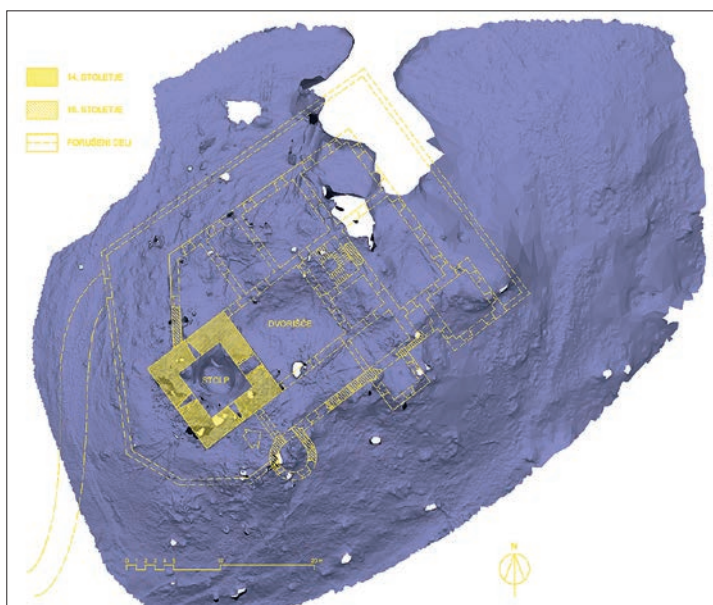
Navpični pogled na ostaline severovzhodnega dela kompleksa gradu Rudenek iz zraka na digitalnem modelu terena ter aplicirana interpretacija tlorisne zasnove gradu s šrafrano označenimi ohranjenimi deli in črtkano označenimi porušenimi deli (posnela in izdelala: Nejc Bernik (UIFS ZRC SAZU) in Igor Sapač, 2024).
