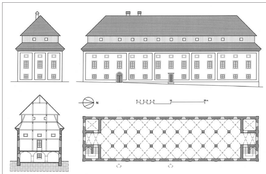
Poskus rekonstrukcije zasnove ojstriške pristave v poznem 18. stoletju. Zgoraj izris stranske južne in glavne vzhodne fasade, spodaj prečni prerez proti severu in tloris pritličja pred vgradnjo predelnih sten med nosilnimi slopi (risal: Igor Sapač, 2017).
