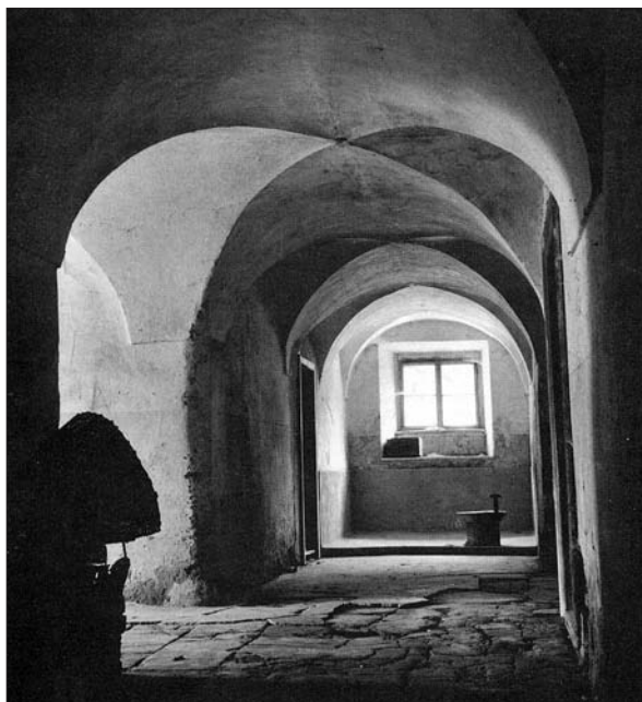
Križno obokani južni del pritličja ojstriške pristave pred rušenjem leta 1964 (ZVKDS OE Celje, objavljeno v: Stopar, Grajske stavbe v vzhodni Sloveniji. Tretja knjiga, str. 96).
