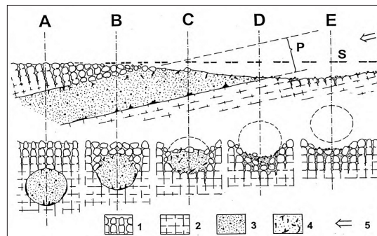
Slika 11: Model nastanka brezstropnih jam.
