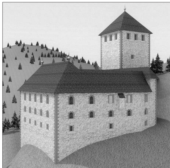
Grad Šoštanj okoli leta 1430. Pogled na grajsko stavbo s severovzhodne strani. Računalniška študija. Poskus rekonstrukcije (izdelal Ivan Tablin na podlagi risb Igorja Sapača, 2021).
